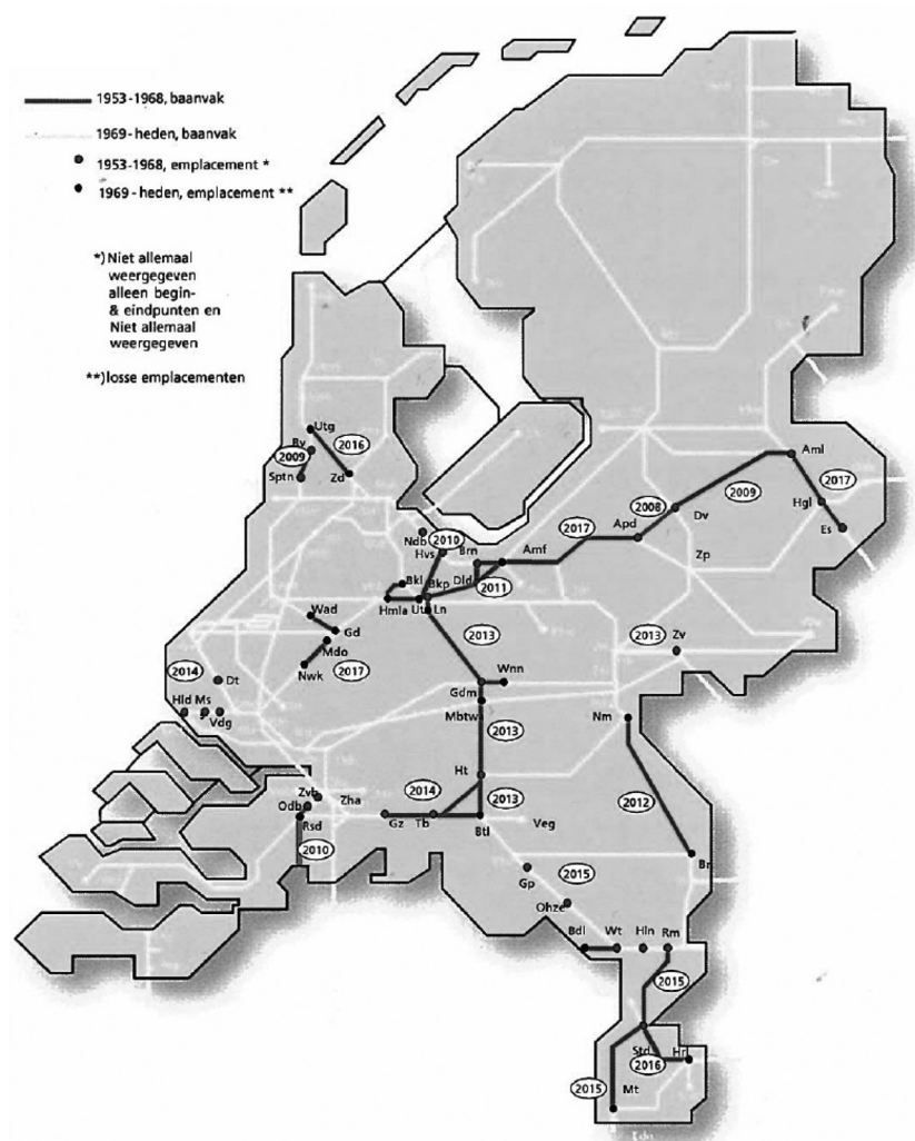
Figuur 17 oorspronkelijke planning vervanging relaisinstallaties '53-'68
